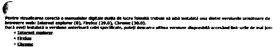
Fig. 2 Actualizare browser
